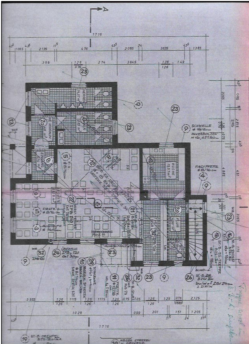
Erdgeschoss
