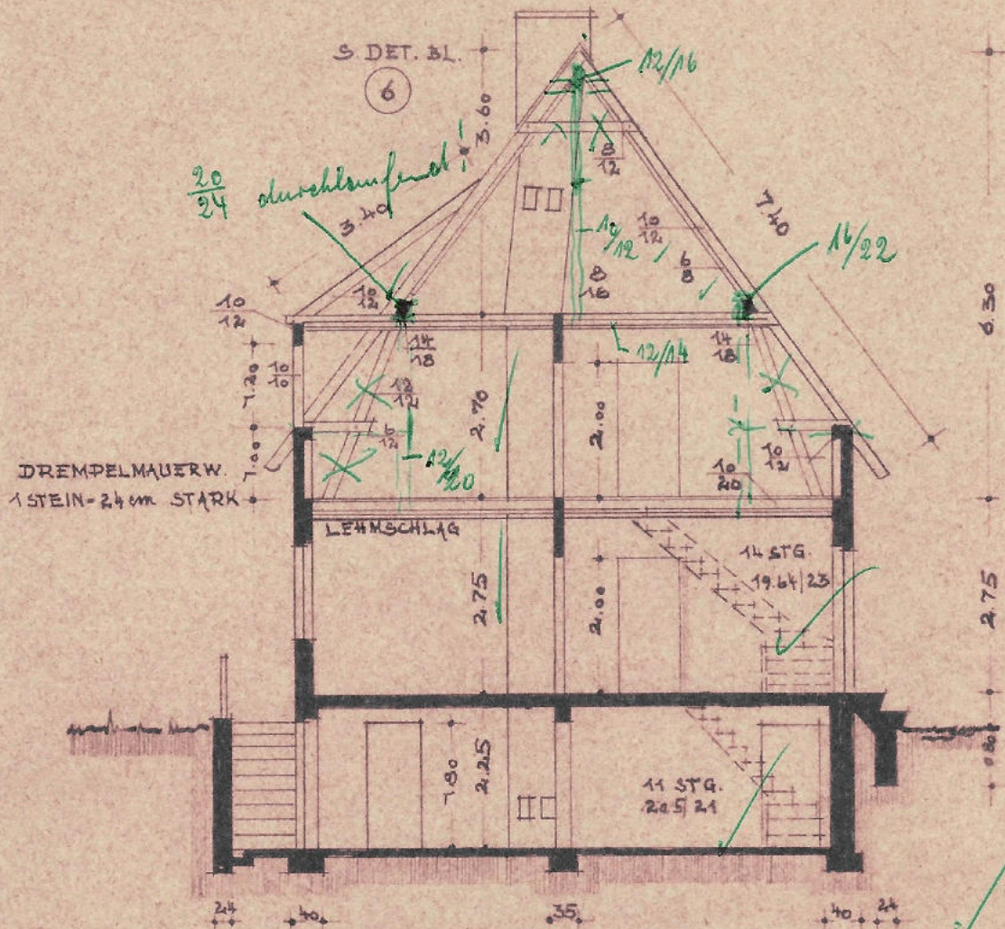
QUERSCHNITT
