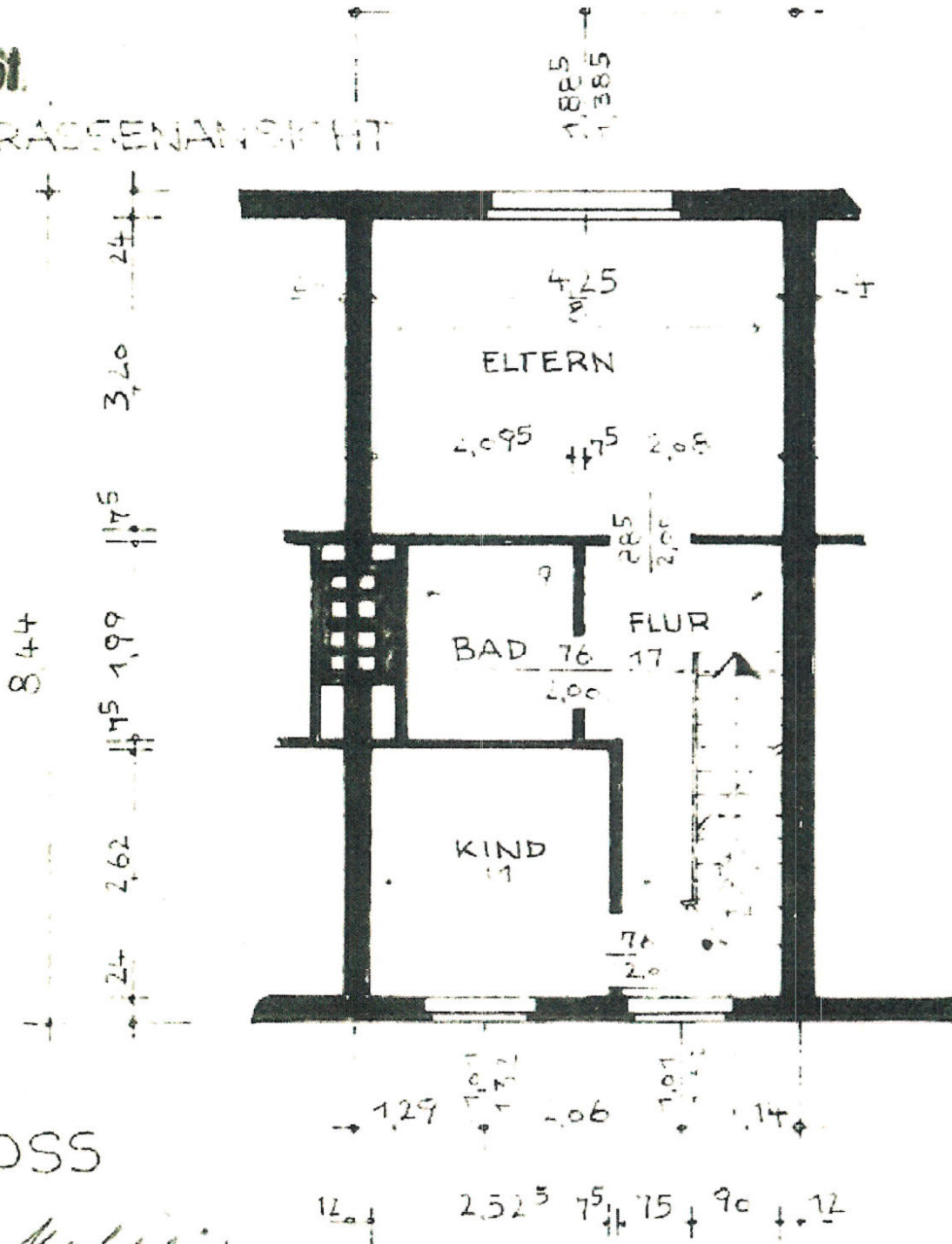
7.2.2 Grundriss Obergeschoss
